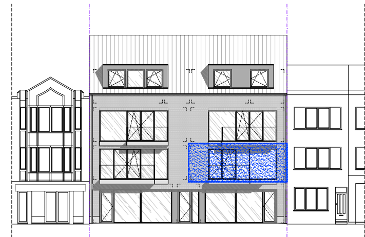
Vorgevel
